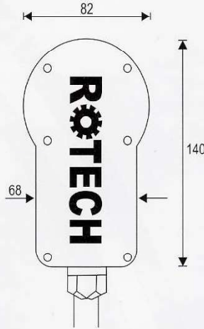
TYPE E2 (P.N.P.) 10 - 30 Vdc
