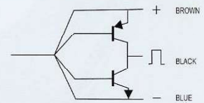
TYPE E3 (P.N.P + N.P.N) 10 - 30 Vdc
